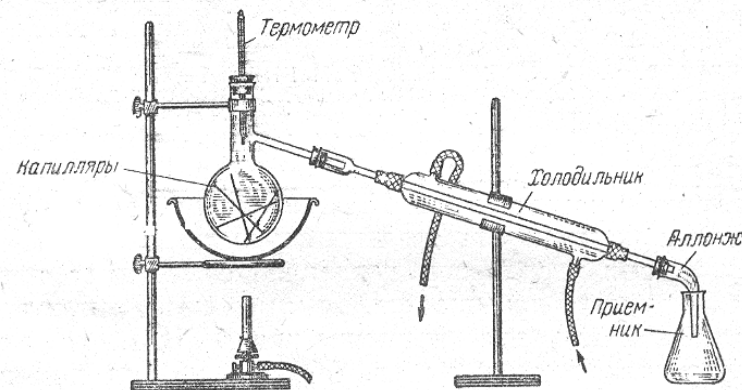
Рис. 1. Установка для перегонки нефти.
